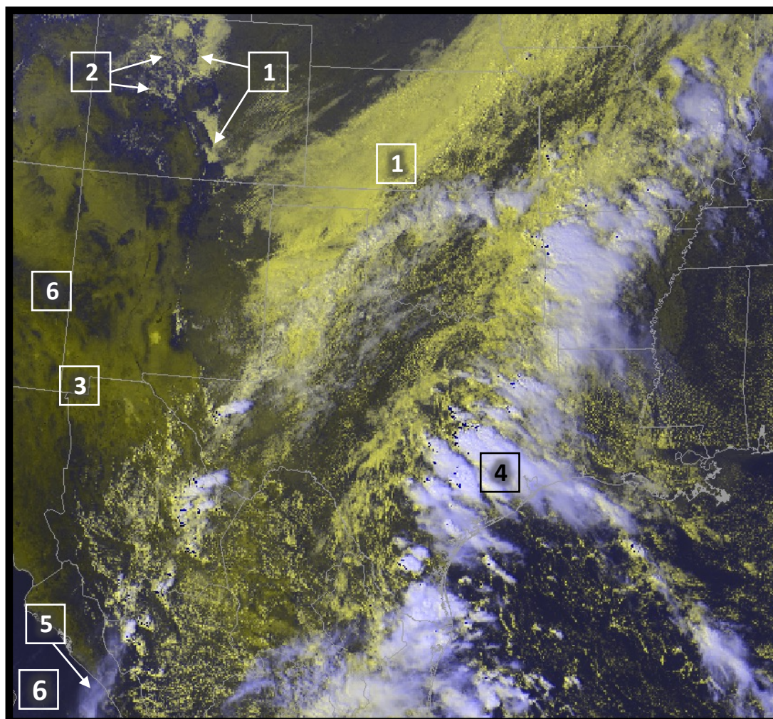
Producto RGB Convección de nubes en el día del ABI GOES-16, 3 octubre 2017 a las 2222 UTC
